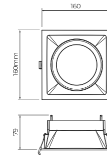
Dimensão do corte: 145x145mm
