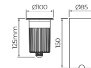
Dimensão do corte: Ø79mm (3 1/8")
