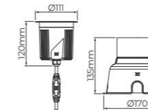
Dimensão do corte: Ø92mm (3.5/8")
