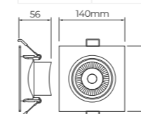
Dimensão do corte: Ø118mm (4,3/4")
