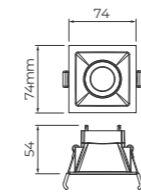
Dimensão do corte: 62x62mm
