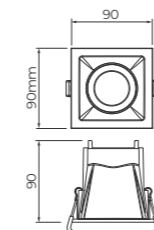
Dimensão do corte: 79x79mm
