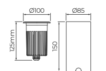
Dimensão do corte: Ø79mm (3,1/8")
