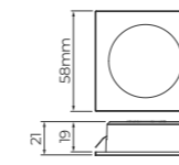
Dimensão do corte: Ø50,8mm (2")
