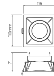
Dimensão do corte: 100x100mm
