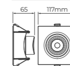
Dimensão do corte: Ø92mm (3,5/8")
