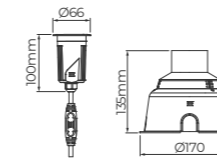
Dimensão do corte: Ø51mm (2")
