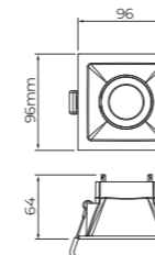
Dimensão do corte: 80x80mm
