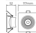
Dimensão do corte: Ø90mm (3,5/8")
