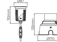
Dimensão do corte: Ø68mm (2.11/16")
