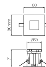
Dimensão do corte: Ø64mm (2.1/2")
