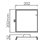
Dimensão do corte: 185x185mm
