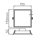
Dimensão do corte: 155x155mm
