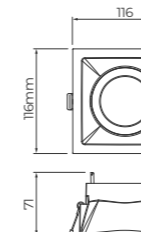
Dimensão do corte: 100x100mm
