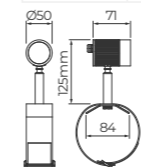
Diâmetro máximo da cinta: Ø130mm
