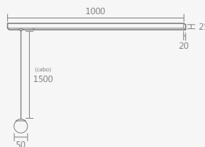
1015 – perfil sobrepор print LED pendente mini globo
