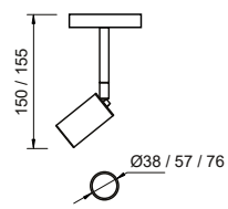
Com canopla
