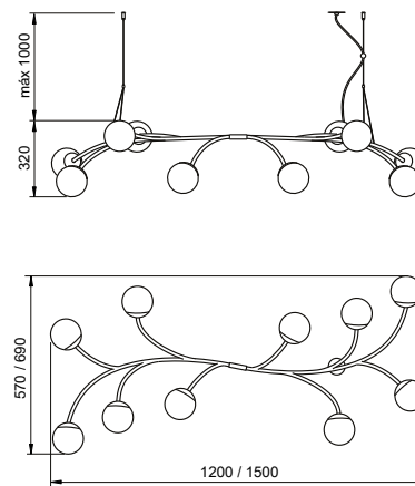
Pendente /6 /10
