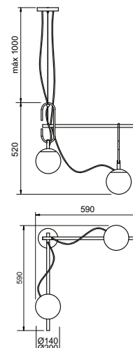
Pendente /2
