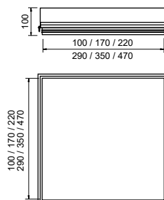
Quadrado
