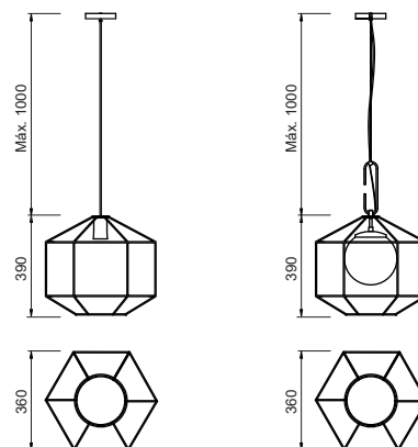
Sem Globo
