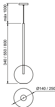
Pendente
