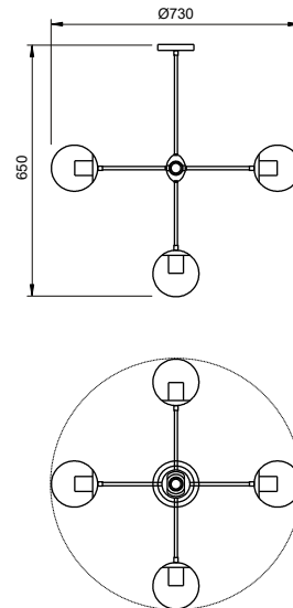
Pendente /4 /5 /6
