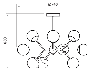
Pendente
