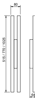
Perfis Alinhados
