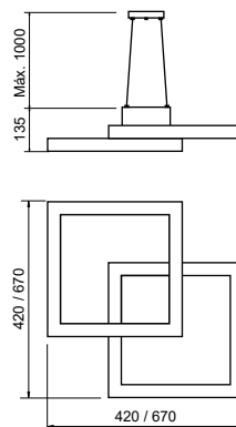
Pendente
