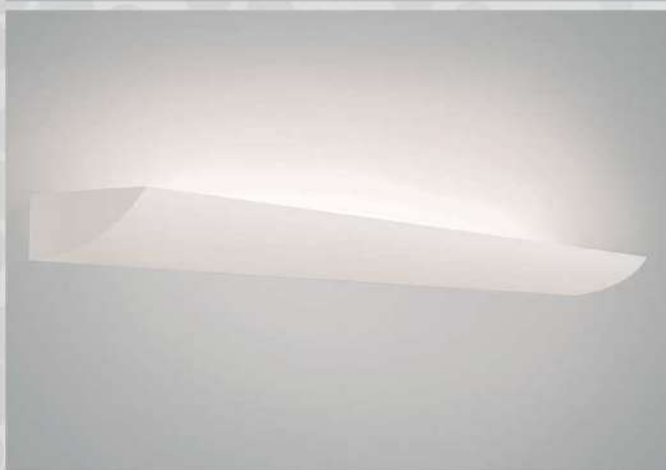
ARANDELA 4036 G Porta lâmpada: 1 x G13 T8 LED Tubular (T8 1200 mm) Luminária: \Leftrightarrow 1245 x \varnothing 70 mm Profundidade: \nearrow 165 mm * Não acompanha lâmpada
