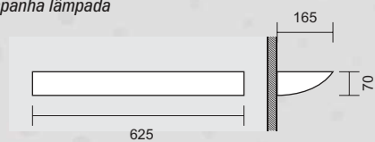
ARANDELA 4036 P Porta lâmpada: 1 x G13 T8 LED Tubular (T8 600 mm) Luminária: \Leftrightarrow 625 x \varnothing 70 mm Profundidade: \nearrow 165 mm * Não acompanha lâmpada
