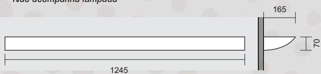
ARANDELA 4036 G Porta lâmpada: 1 x G13 T8 LED Tubular (T8 1200 mm) Luminária: \Leftrightarrow 1245 x \varnothing 70 mm Profundidade: \nearrow 165 mm * Não acompanha lâmpada
