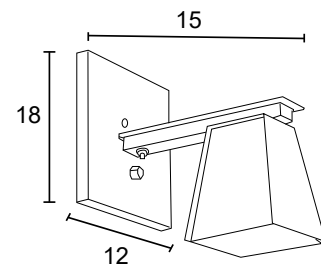
AE 237 IP54 – Indicado para uso externo 1x Alumínio Medidas em cm
