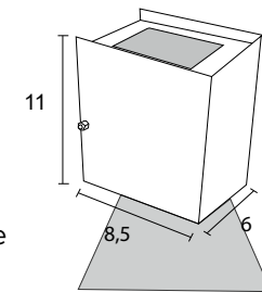
AE 107 IP54 – Indicado para uso externo 1x Alumínio e vidro transparente Medidas em cm
