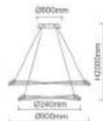
DCD00789 Pendente D600+800° H2000mm Dourado 80W Alumínio e Cristal Bivolt
