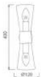
Tulipa DCB00281 Arandela Metal+Vidro Bronze Ø120*400mm E14*2
