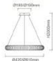
DCD00786 Cromado 43W Ø420*H2000mm DCD00787 Cromado 65W Ø460*H2000mm Pendente Alumínio e Acrílico Bivolt
