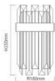
DCB00219 Arandela Metal+cristal Dourado 180*330mm E14*2
