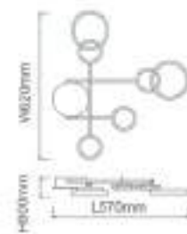
DCB015093 Arandra 620*570mm Dourado LED 23W Alumínio e Silicone Bivolt
